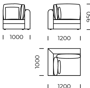
Siedzisko narożne B / Corner seat B
