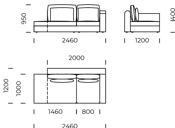
Tapczan lewy B2 / Left couch B2
