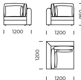
Siedzisko narożne C / Corner seat C
