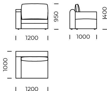
Siedzisko lewe B1 Left seat B1
