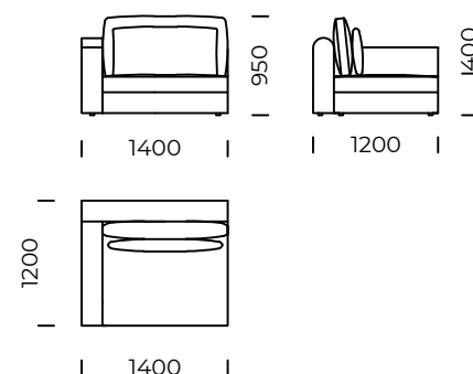
Siedzisko narożne C / Corner seat C
