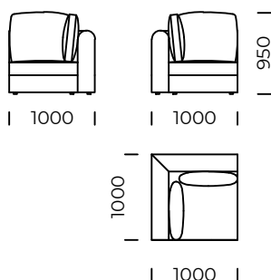
Siedzisko narożne A / Corner seat A
