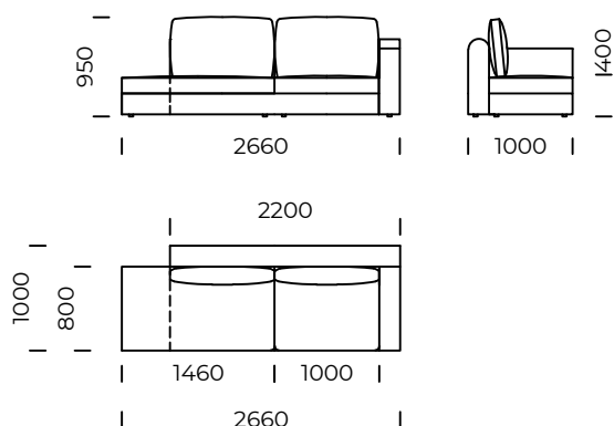
Tapczan lewy B1 / Left couch B1
