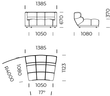
Siedzisko łukowe 1 / Curved seat 1
