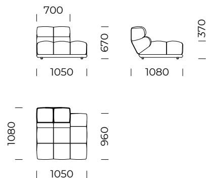
Półwysep prawy / Right Backrest sofa module
