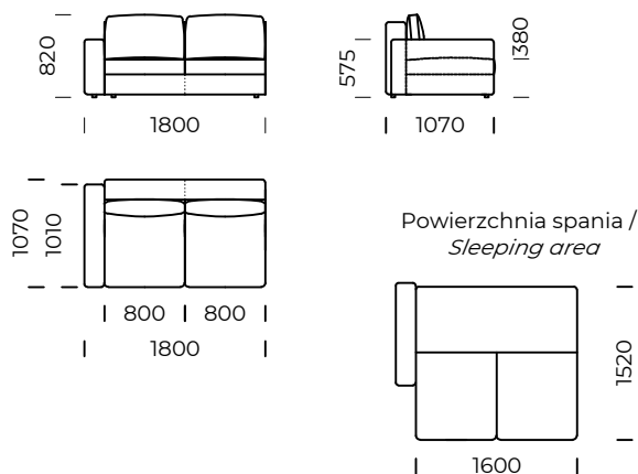
Siedzisko lewe B1 / Left seat B1
