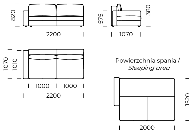
Siedzisko lewe B2 / Left seat B2
